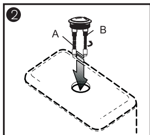
A) nastaviteľná tyč / nastaviteľná tyč / adjustable rod / verstellbarer Stab / tige réglable / varilla ajustable / verstellbare stang / asta regolabile / tija reglabilă / állítható rúd / przęt regulacyjny
