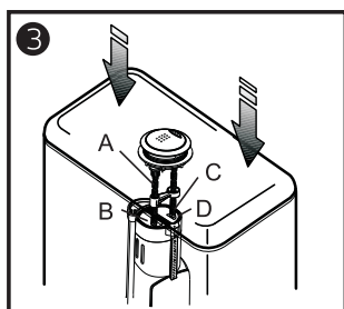
A) černá tyč / čierna tyč / black rod / schwarzer Stab / tige noire / varilla negra / zwarte stang / asta nera / tija roșie / fekete rúd / czarny przęt
