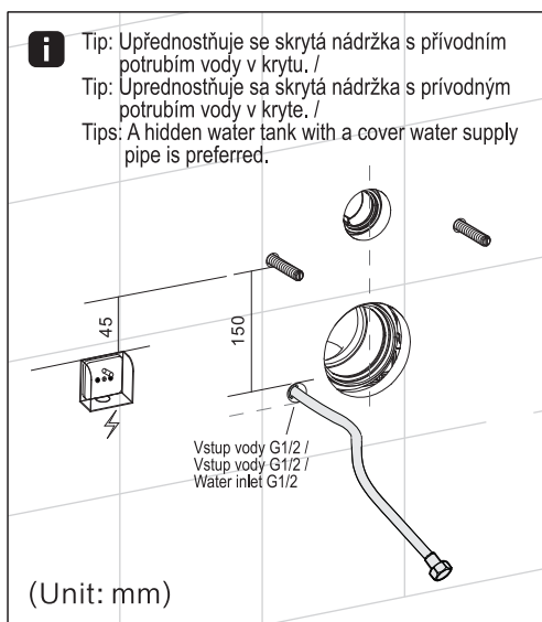
Nákres dokončené instalace / Náčrt dokončenej inštalácie / Installation complete sketch
